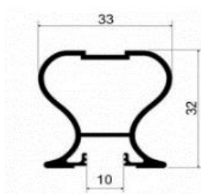
Senator (алюминий) - Закрытый тип MS 110
