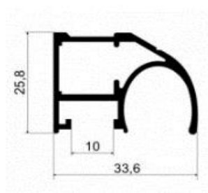
Senator (алюминий) - Открытый тип MS 120
